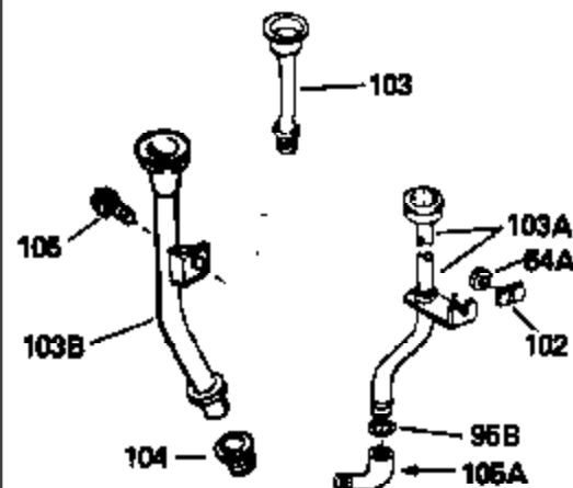
STD. POINT
